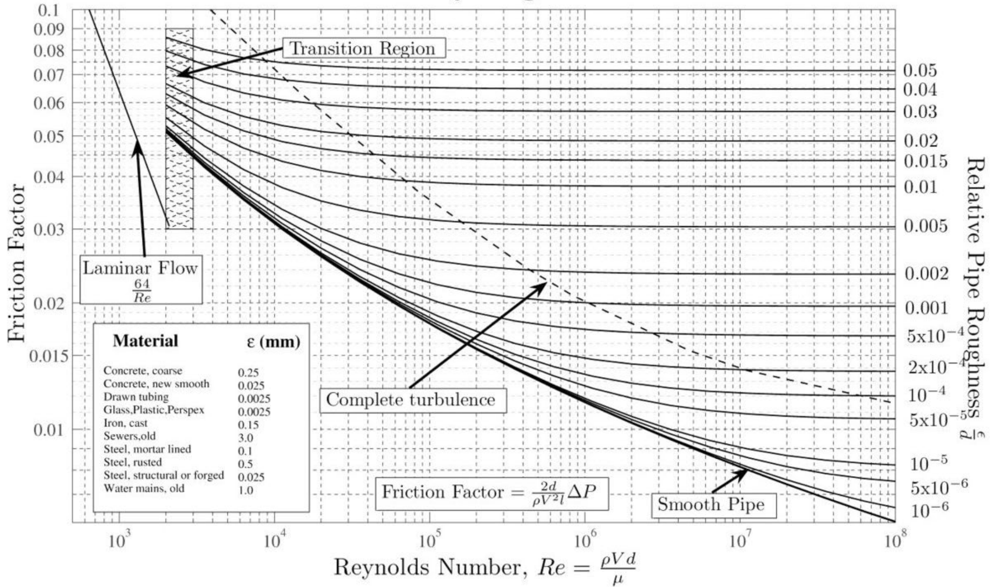
Διάγραμμα Moody
