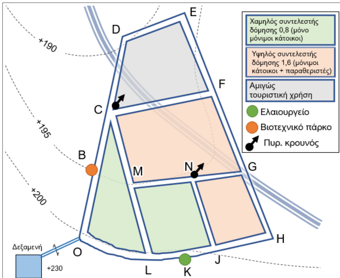
Σχήμα 2: Κάτοψη οικισμού.
