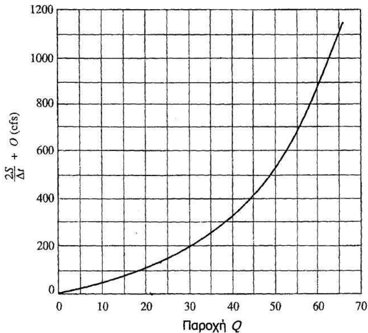
Σχήμα 7.12 Σχέση παροχής Q και 2S/\Delta t + Q .
