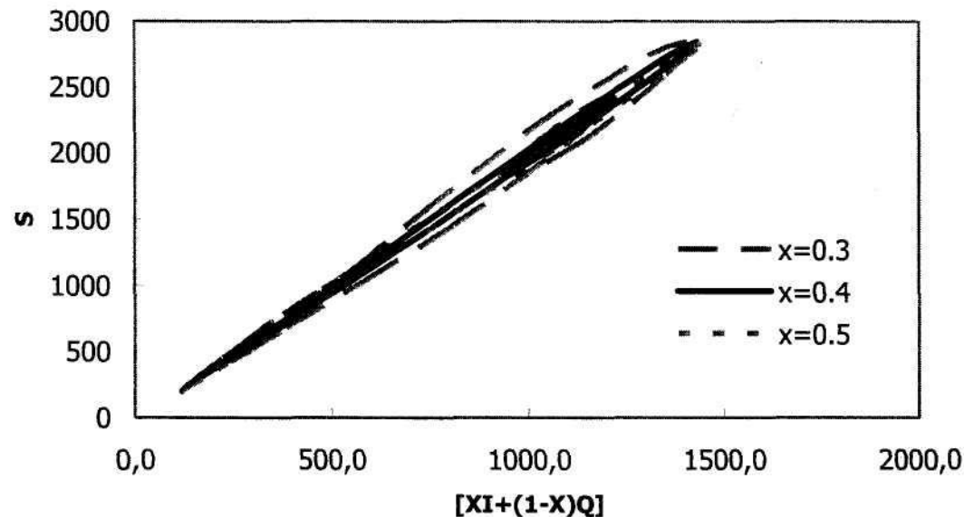
Σχήμα 7.8 Εύρεση της πιο κλειστής αναδιπλούμενης καμπύλης για διάφορες τιμές του x
