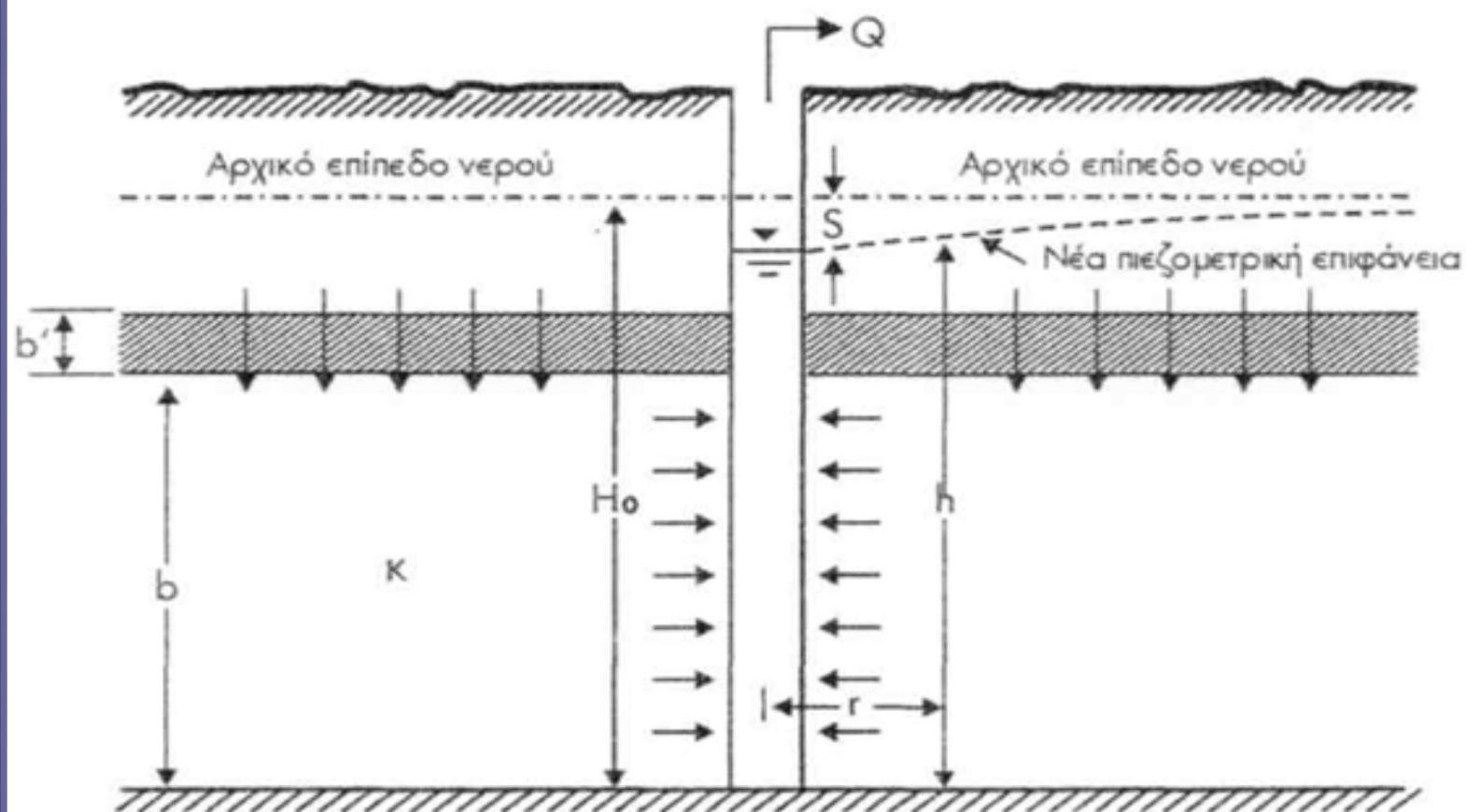
Σχήμα 6.5 Ημιπεριορισμένος υδροφόρας.
