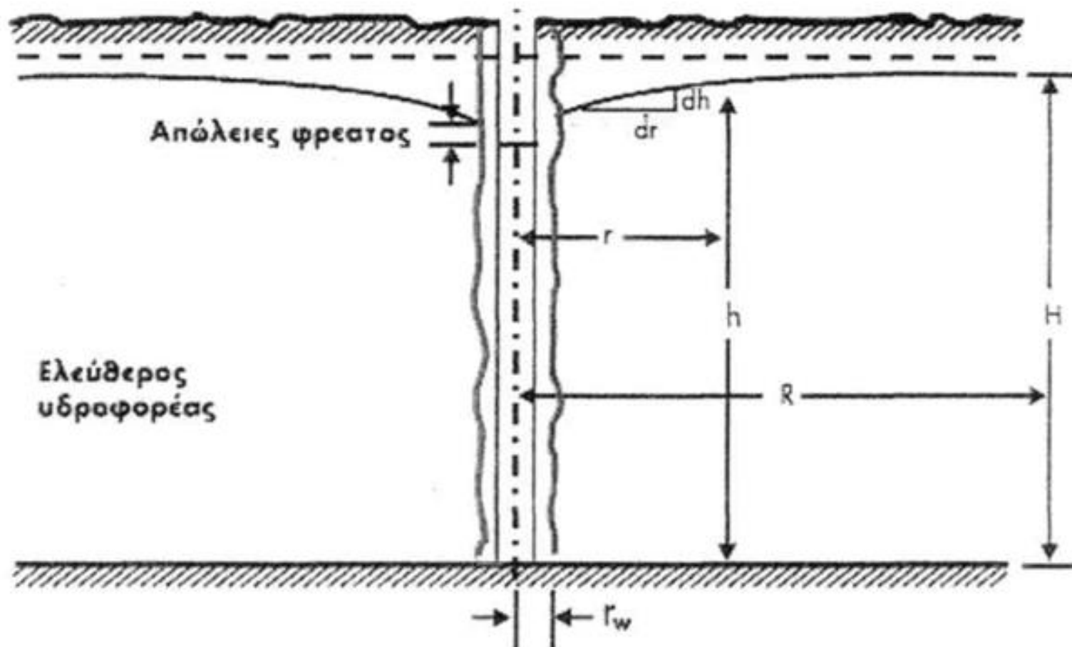
Σχήμα 6.4 Ελεύθερος ή φρεάτιος υδροφόρας.
