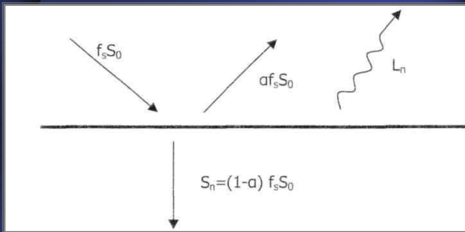
Σχήμα 3.2 Ενεργειακό ισοζύγιο σε υδάτινη ή εδαφική επιφάνεια.
