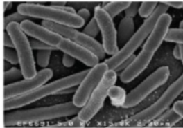
Bacillus
